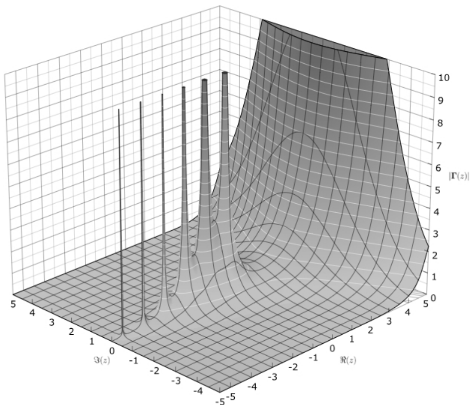
Module de la fonction gamma sur le plan complexe
